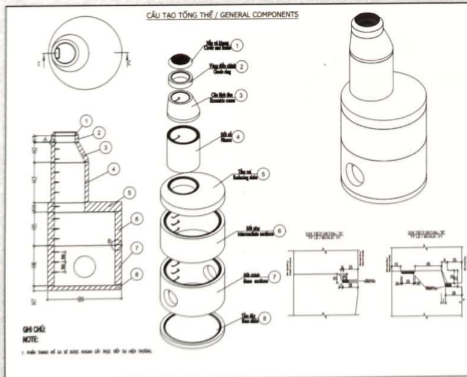
HỐ GA TRÒN LẮP GHEP THEO TIÊU CHUẨN TCVN 10333-4:2019
